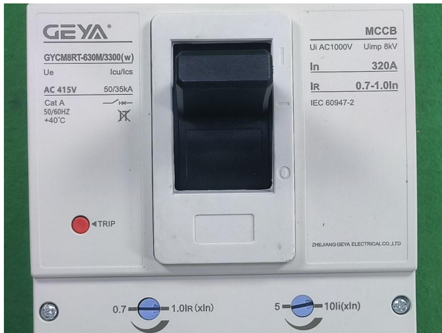
GYCM8RT-630M/3300(w), 320 A, 3P
